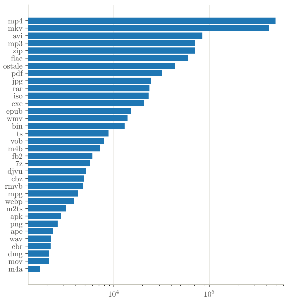
Slika 5.2: Tipi glede na število torrentov, pri katerih tip predstavlja glavno velikosti.
